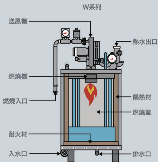
熱水鍋爐內部構造
